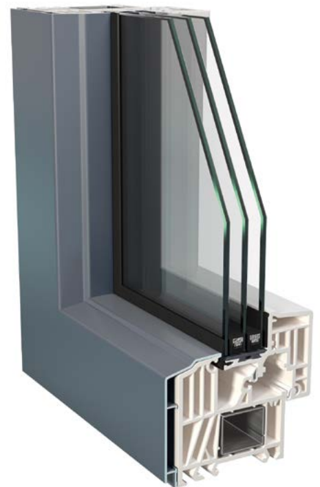
EMO Novaline mit optionaler 3-fach Verglasung
